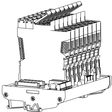
安装示意图
